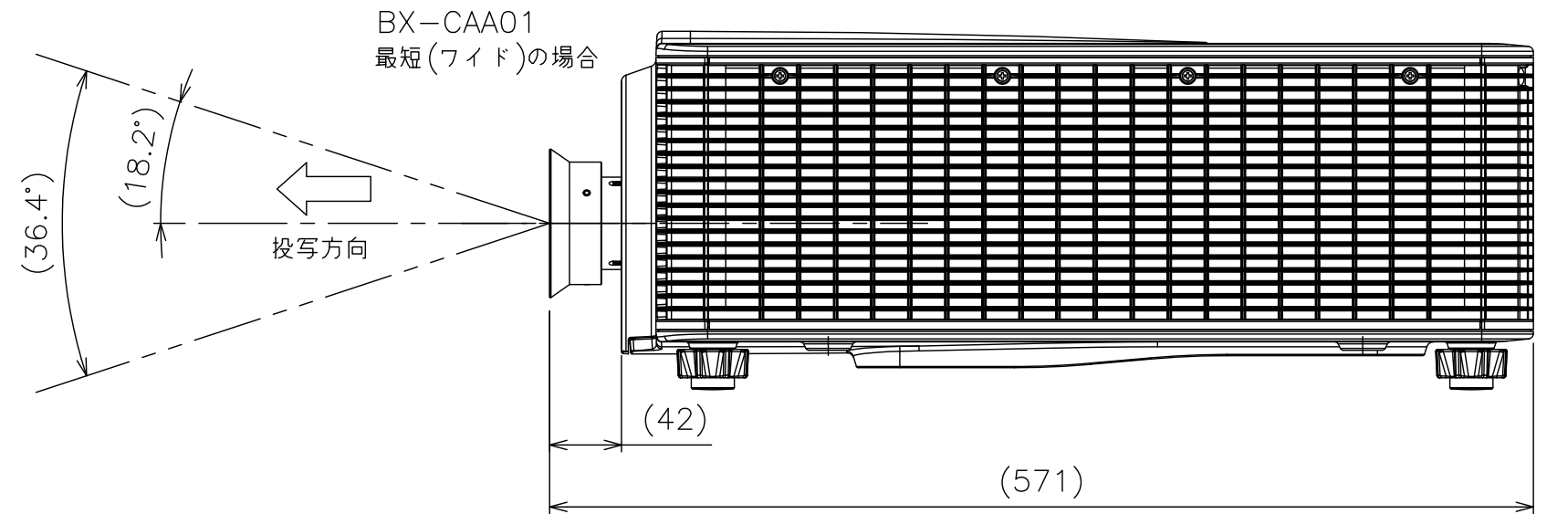
ZU1300装着時寸法(S=1:4)
