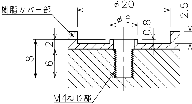
プロジェクター取付穴詳細図
