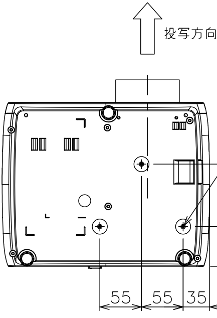
プロジェクター取付穴 3×M4 深さ8
