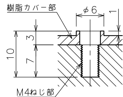
プロジェクター取付穴詳細図
